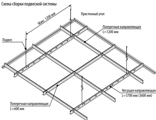
Схема сборки подвесной системы
